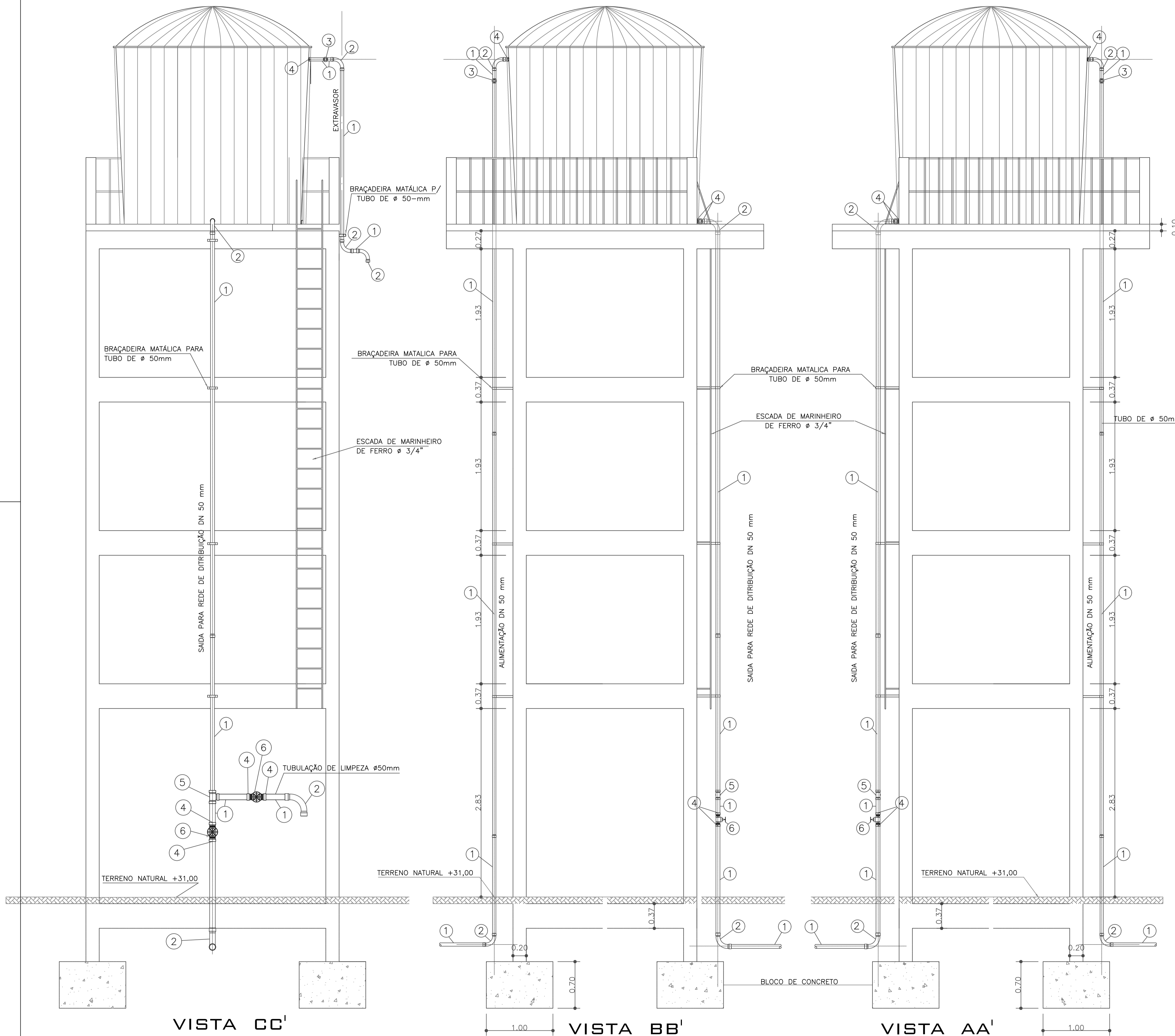
RESERVATÓRIO CAP. 15.000 L
