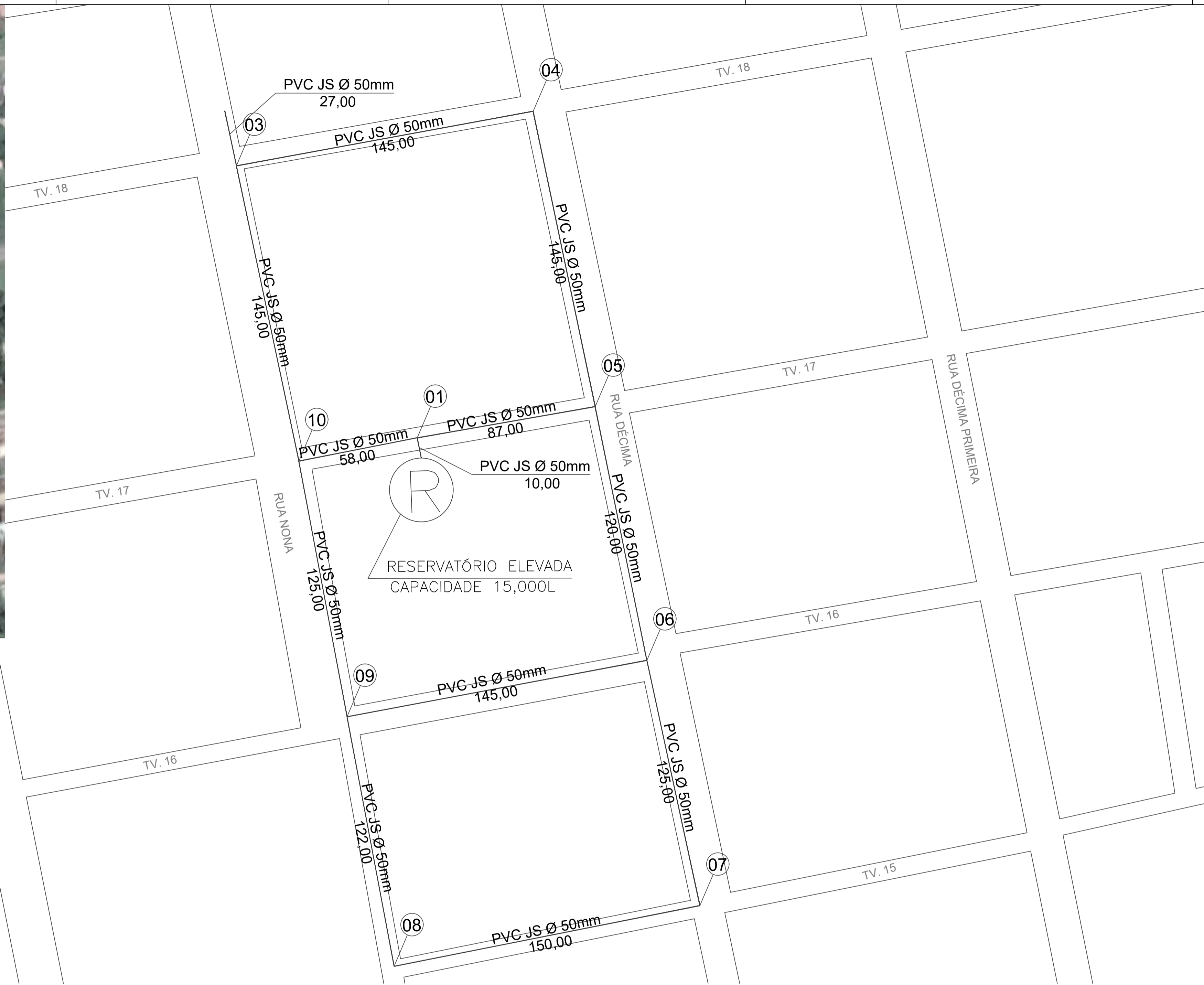
PLANTA DE LOCALIZAÇÃO DA REDE
