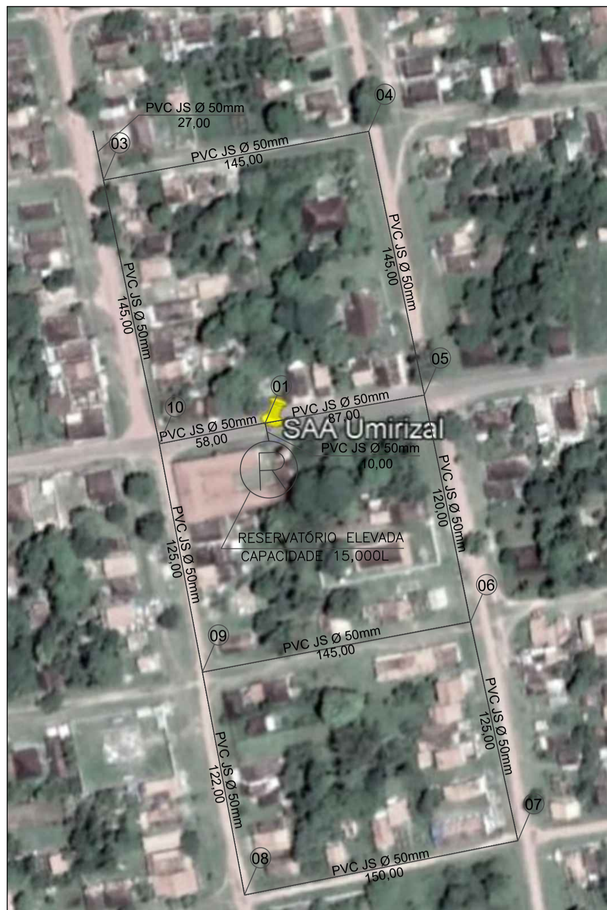
PLANTA DE LOCALIZAÇÃO DA REDE
