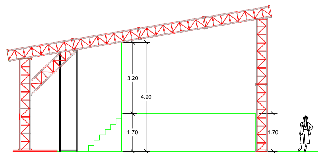
VISTA LATERAL
