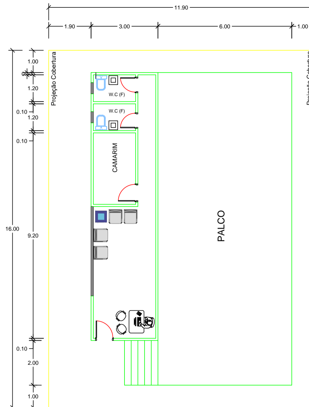
PLANTA BAIXA
