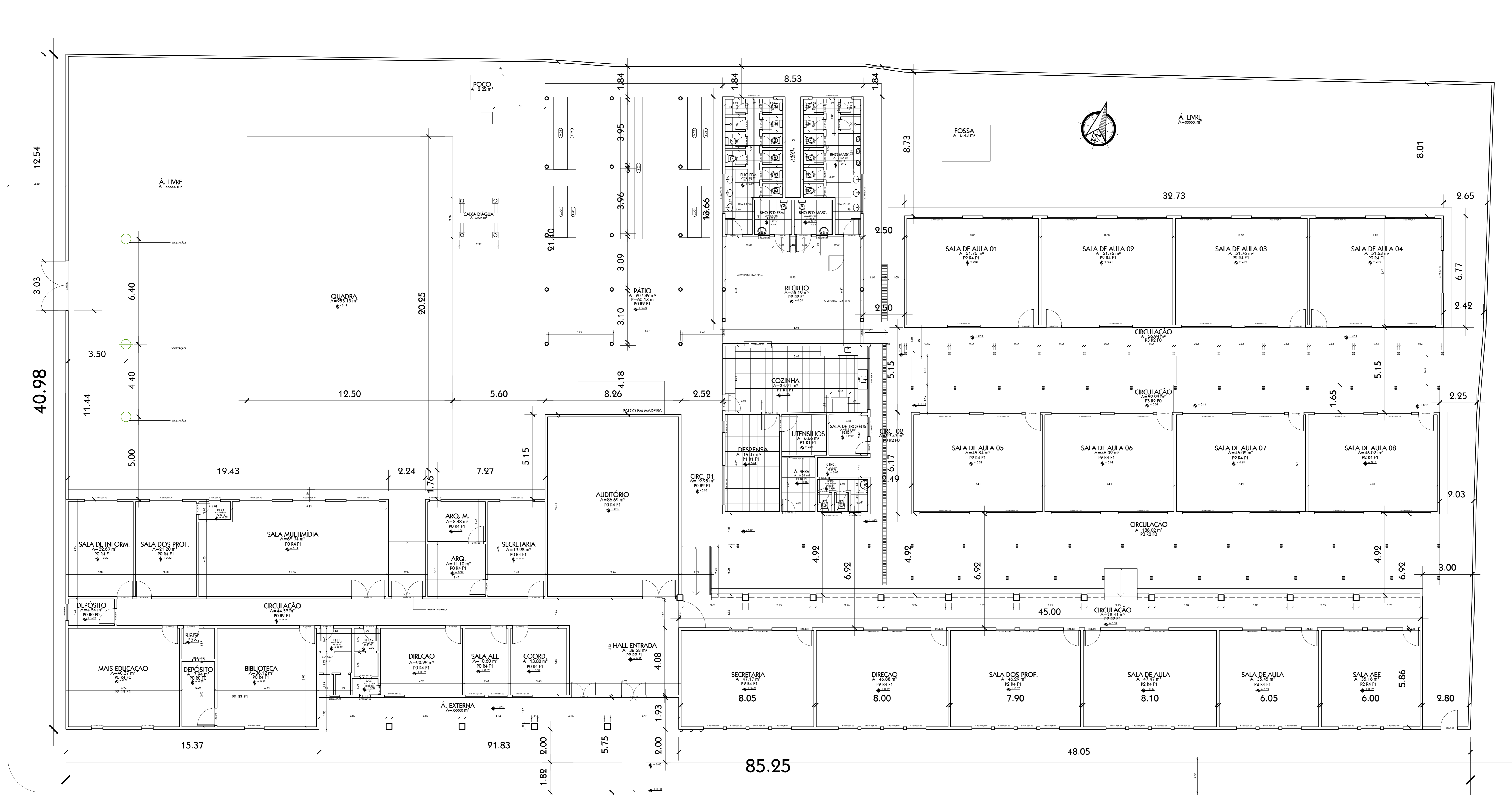
PLANTA BAIXA - EXISTENTE escala.....1:100
