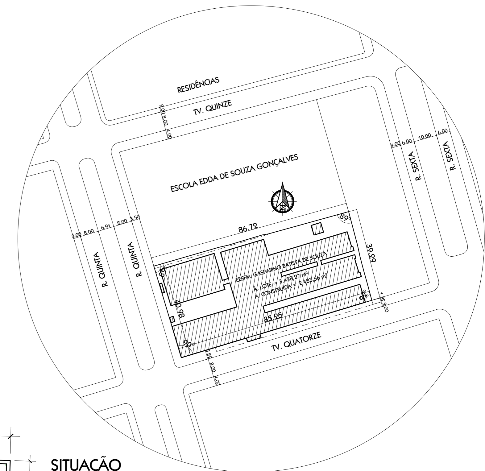
SITUAÇÃO Escala: 1:1000
