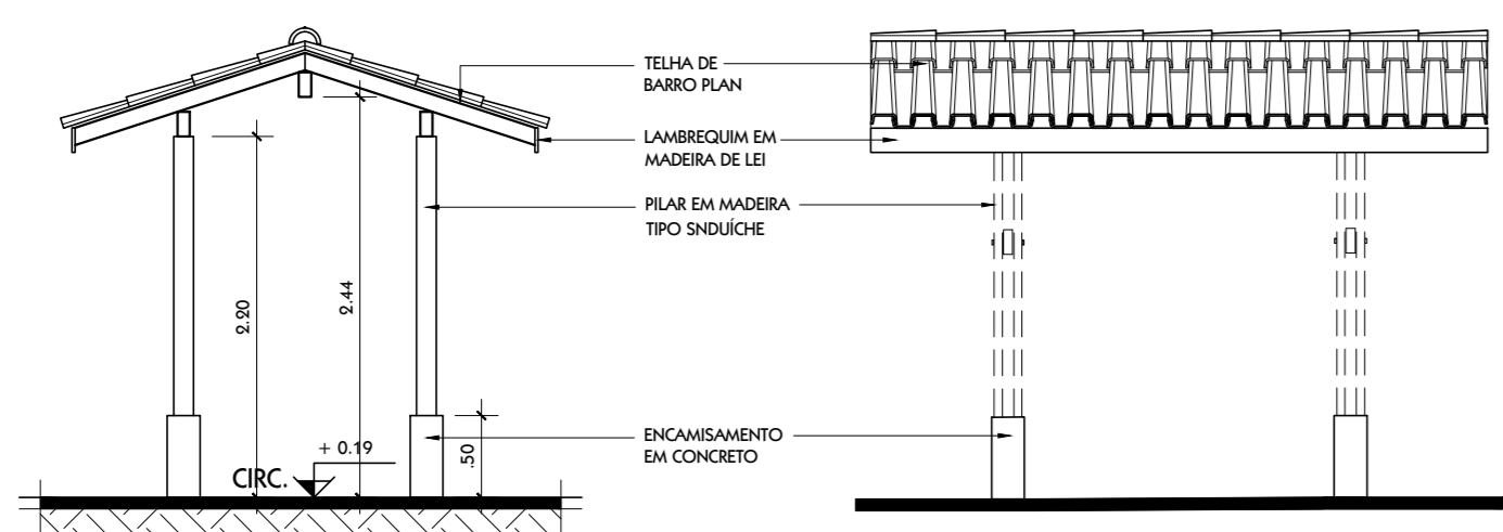
DET. PASSARELA 02 - CORTE escala.....1:50
