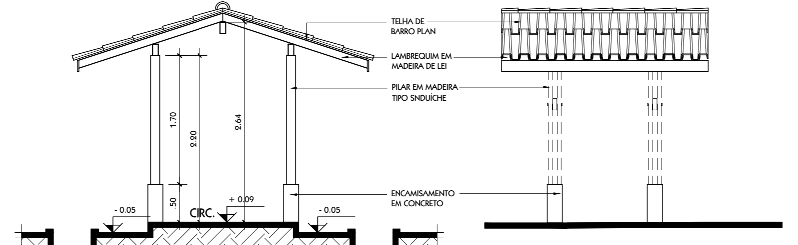
DET. PASSARELA 03 - CORTE escala.....1:50
