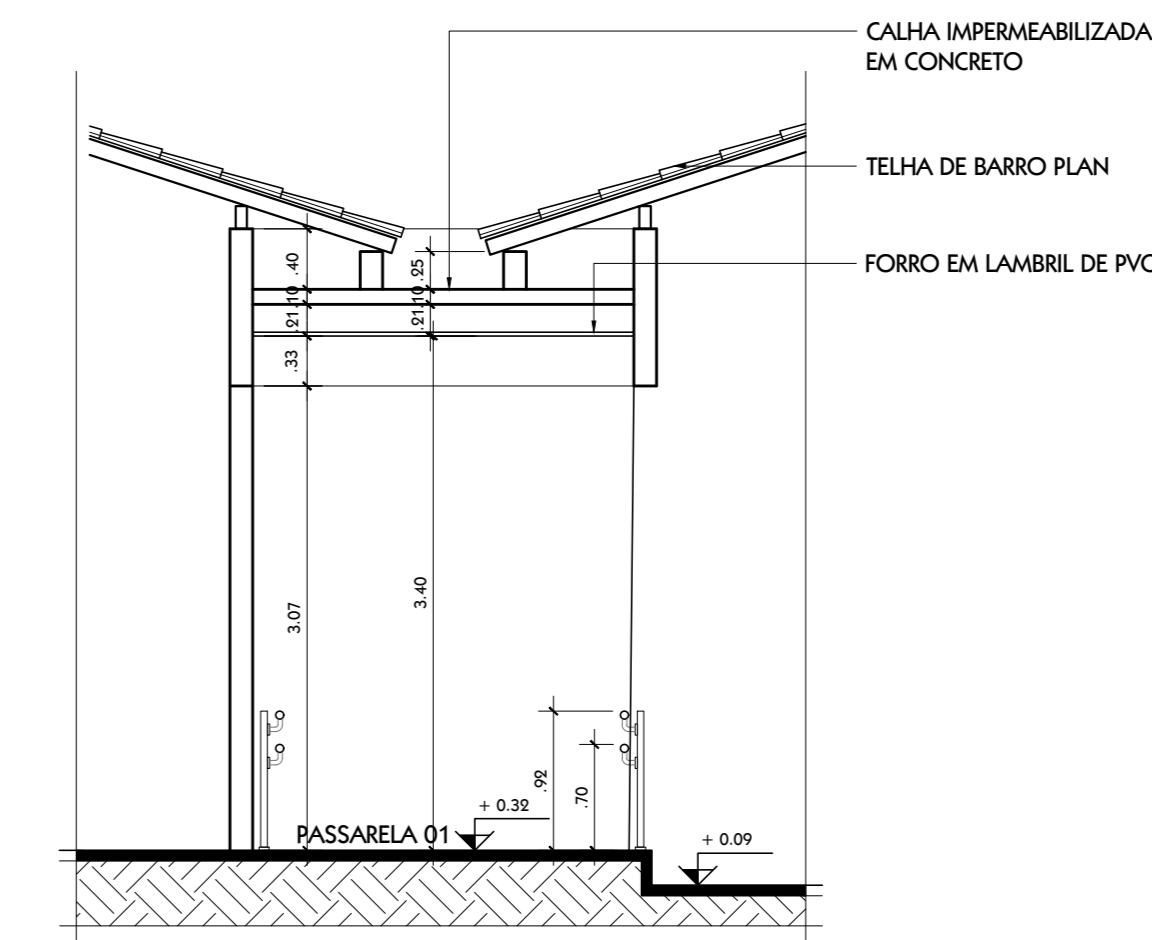
DET. PASSARELA 01 - CORTE escala.....1:50
