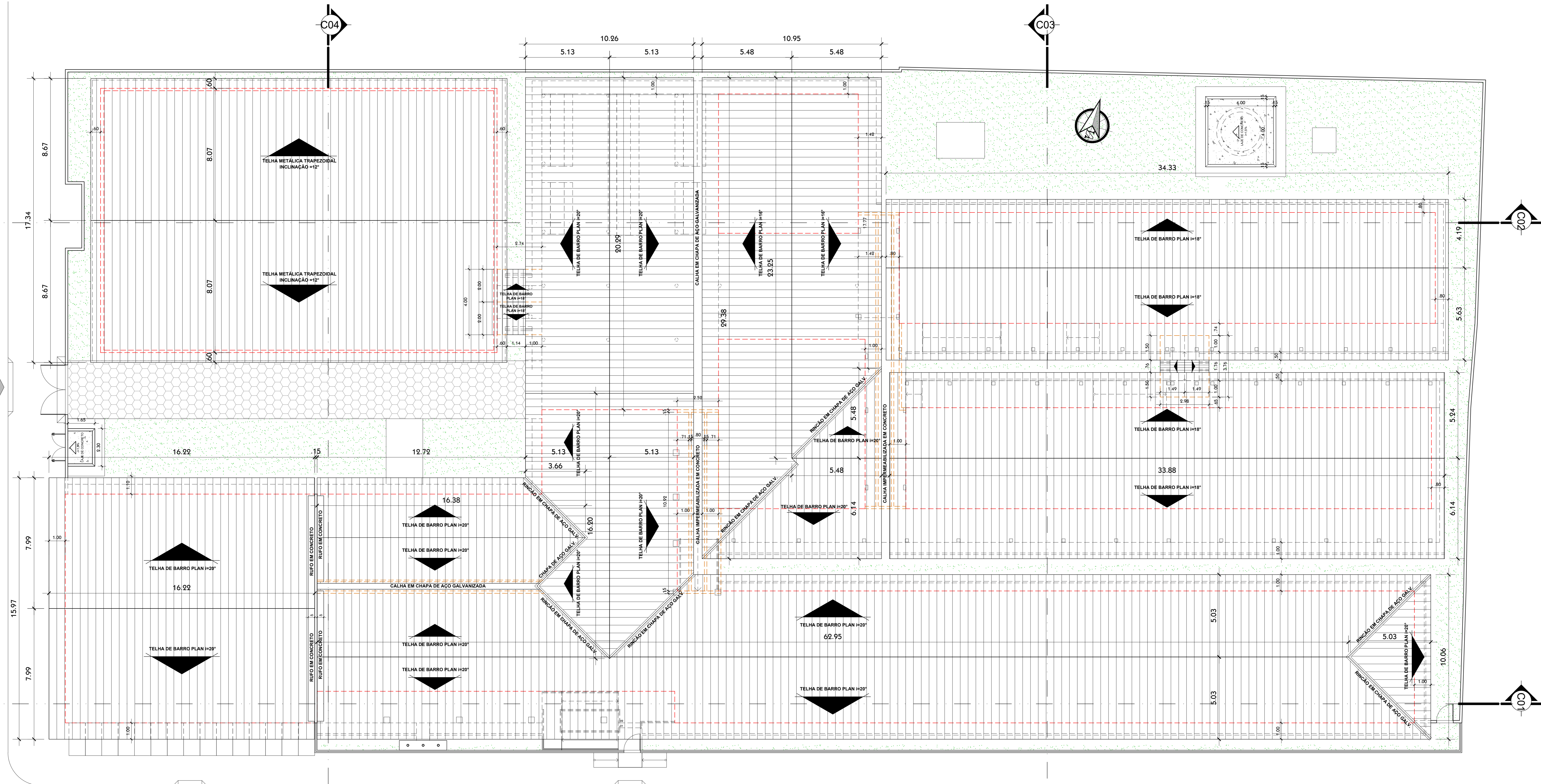
PLANTA DE COBERTURA escala.....1:100
