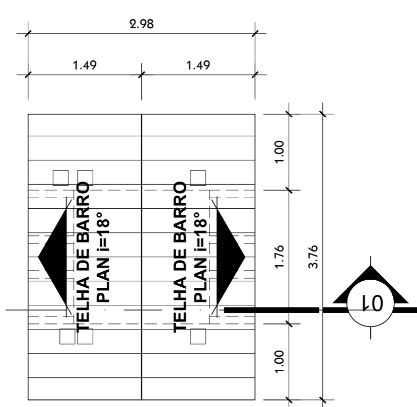
DET. PASSARELA 02 - COBERTURA escala.....1:50
