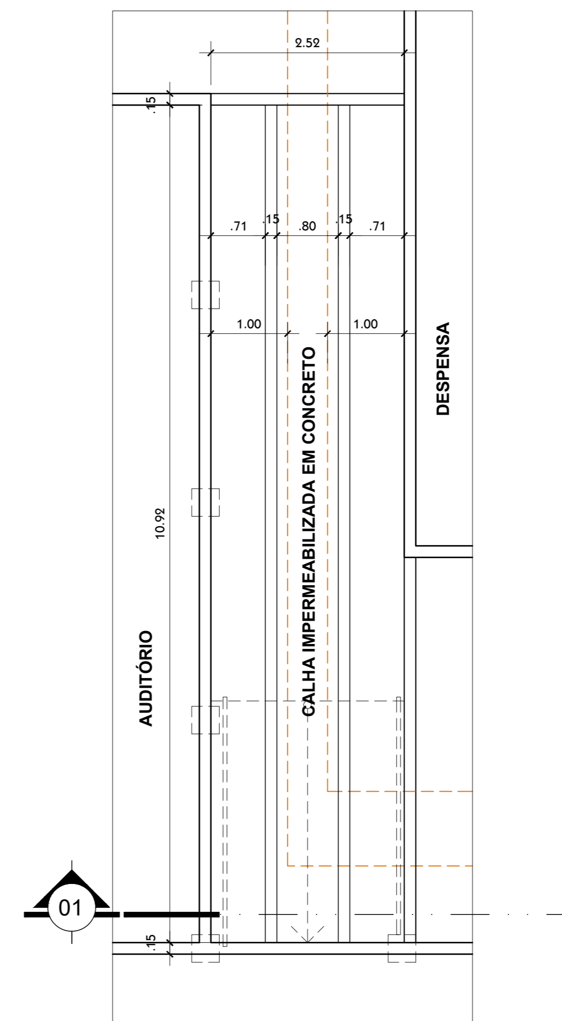
DET. PASSARELA 01 - PLANTA BAIXA escala.....1:50
