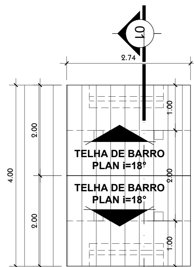
DET. PASSARELA 03 - COBERTURA escala.....1:50
